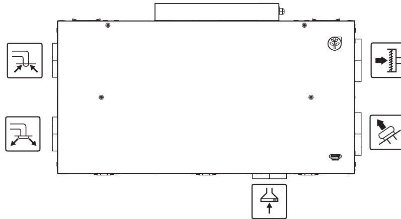
Fig. 2 Kanalanslutningar
