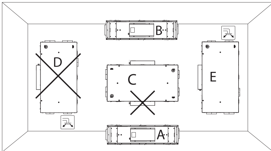
Fig. 3 Möjliga installationspositioner
