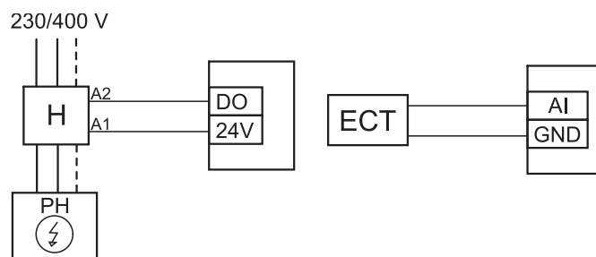
Fig. 13 Fövärmanslutningar
