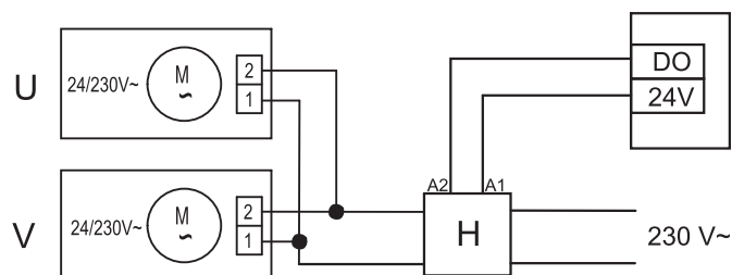
Fig. 17 Spjällanslutning
