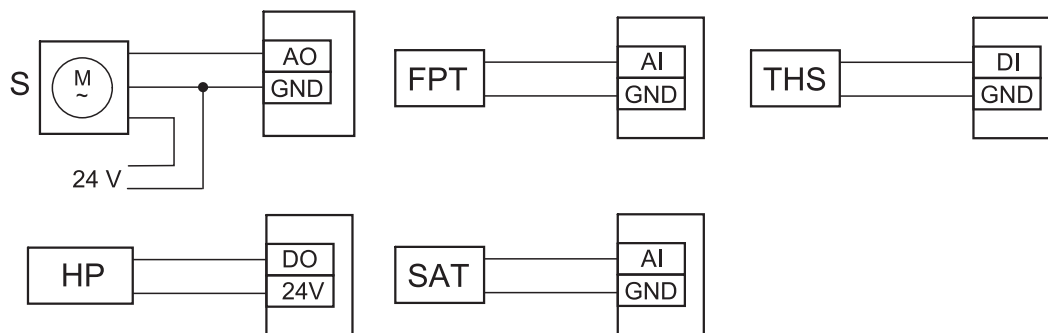
Fig. 16 Växlande uppvärmnings-/kylningsanslutningar
