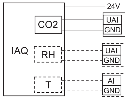
Fig. 12 IAQ-anslutningar
