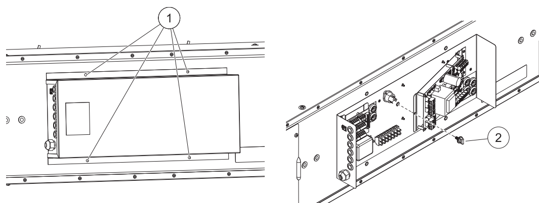
Fig. 4 Kretskort
