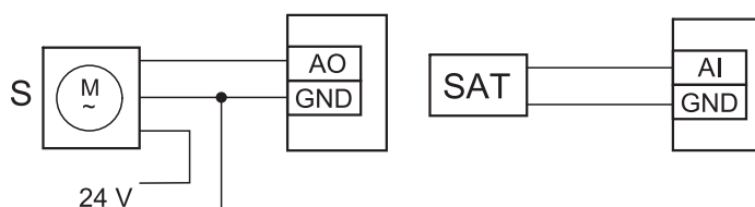
Fig. 15 Kanalkylaranslutningar
