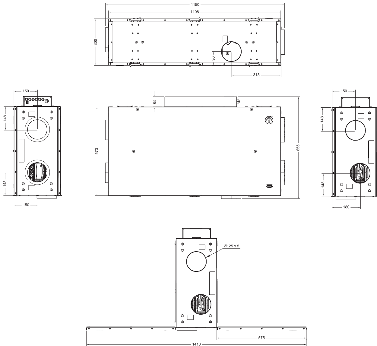
Fig. 1 Mått
