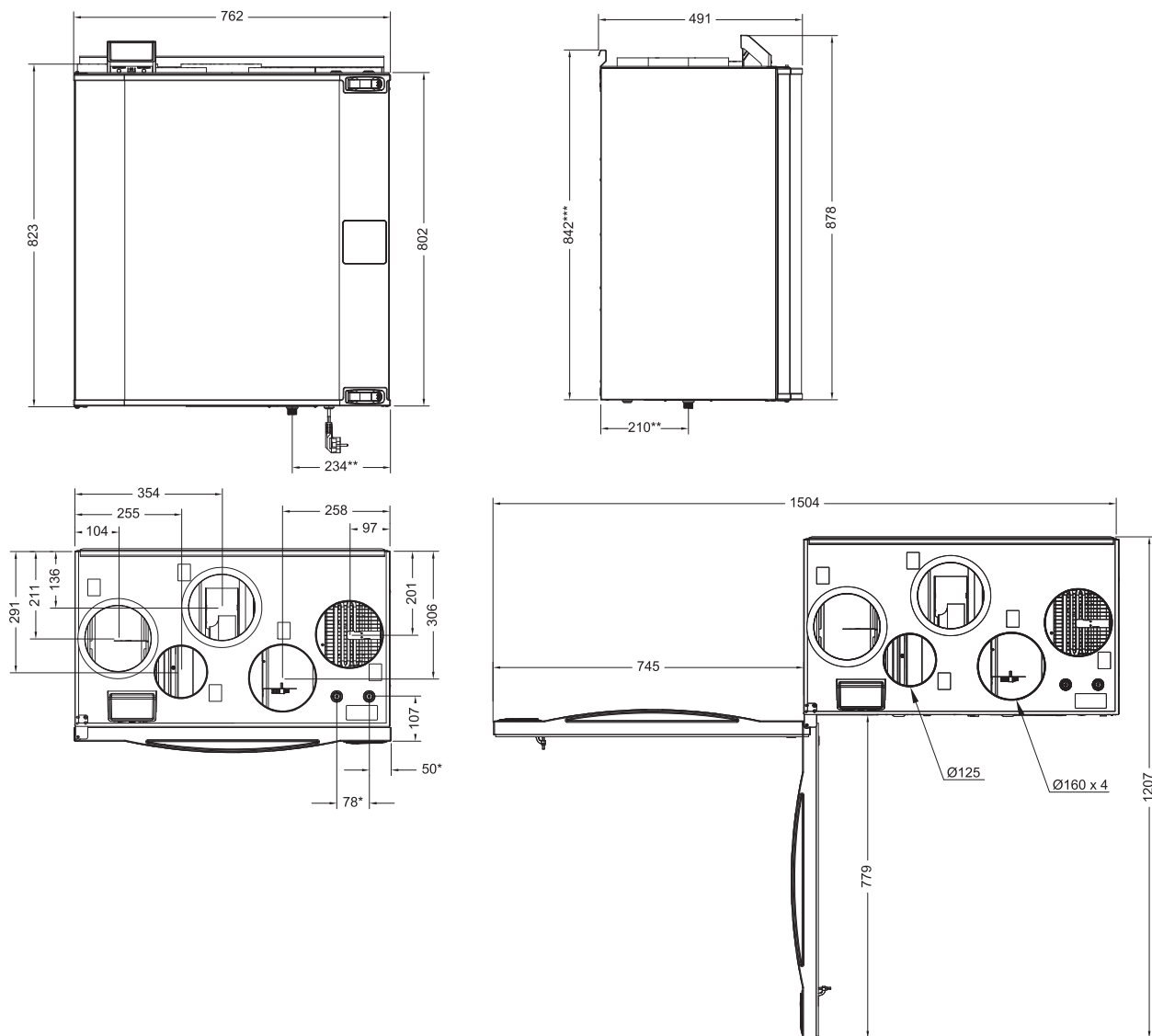
Fig. 2 Mått av högeranslutet aggregat
