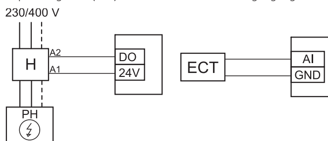
Fig. 14 Fövärmaranslutningar
