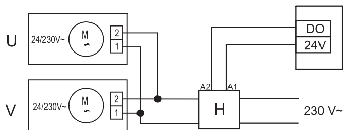
Fig. 19 Spjällanslutning
