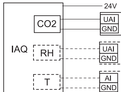
Fig. 13 IAQ-anslutningar
