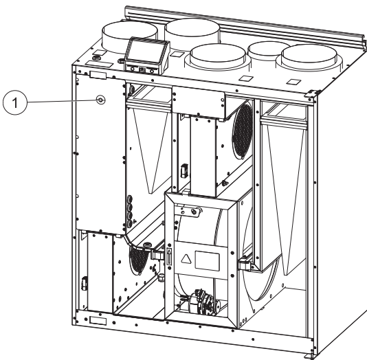
Fig. 11 Återställningsknapp för överhettningsskydd
