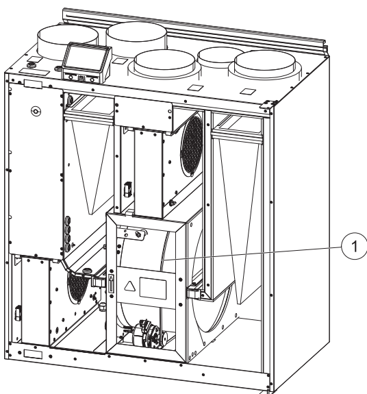
Fig. 12 Rotordrivrem
