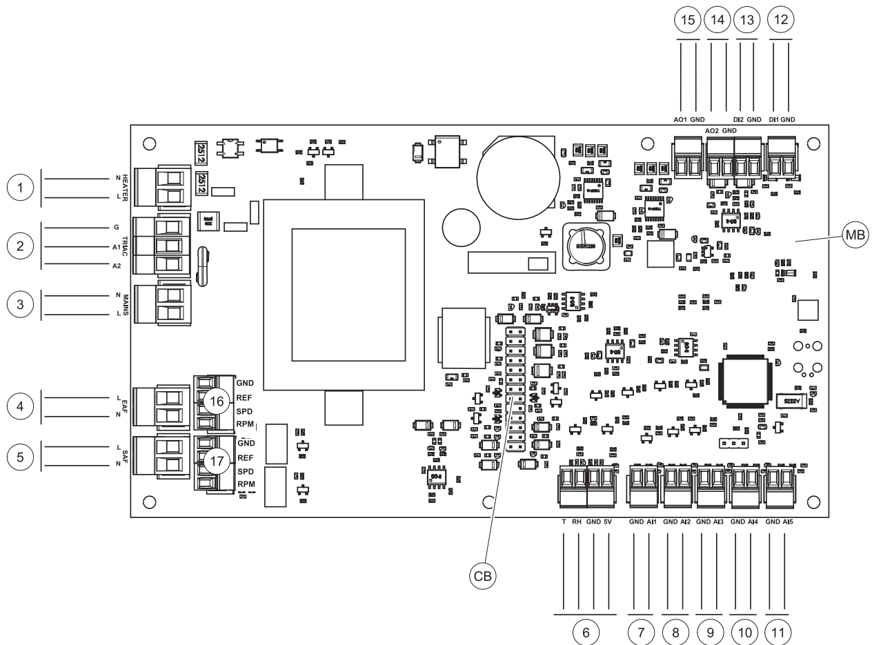
Fig. 8 Huvudkretskortet anslutningar
