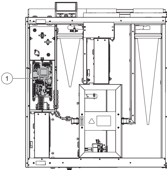
Fig. 7 Kretskortets placering
