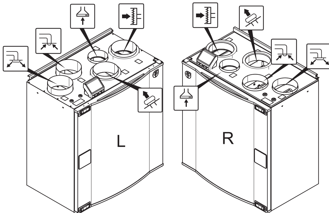
Fig. 3 Kanalanslutningar
