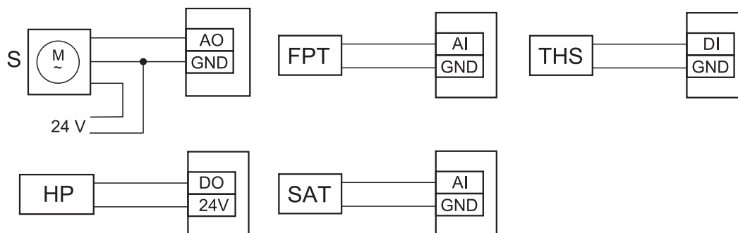
Fig. 18 Växlande uppvärmnings-/kylningsanslutningar
