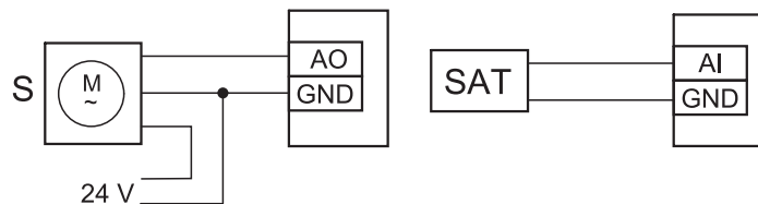
Fig. 17 Kanalkylaranslutningar
